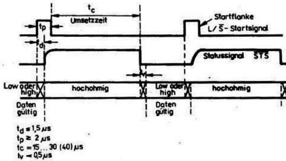
Bild 4: Impulsdiagramm
