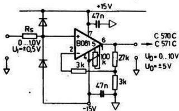
Bild 3: Hochohmiger Vorsatzoperationsverstärker mit Eingangsschutzschaltung
