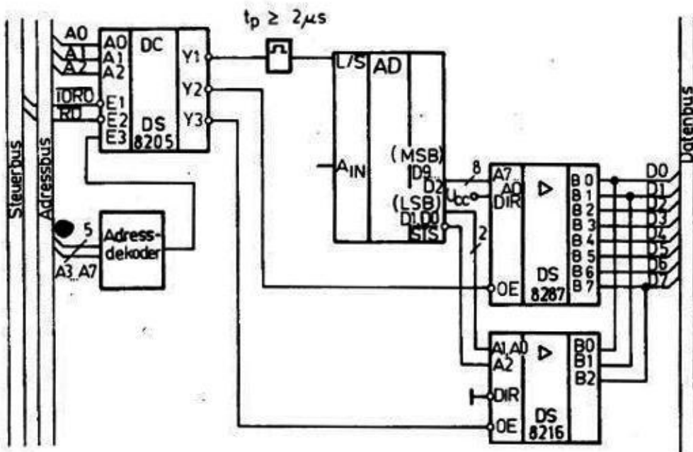
Bild 7: Mikrorechneranpassung (8 bit - Datenbus)
