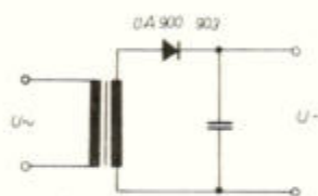
Schaltungsbeispiel für Si-Universaldioden OA 900...903 Gleichrichtung von Wechselspannungen kleiner Leistungen (250 mW)
