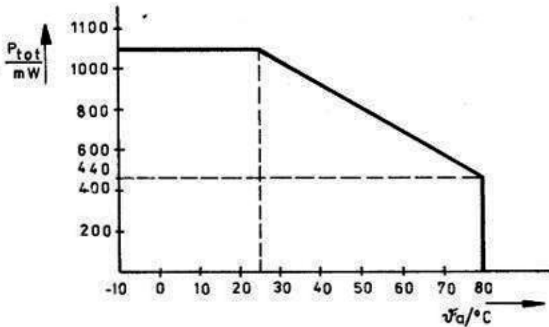
Bild 3: Verlustleistungsreduktionskurve
