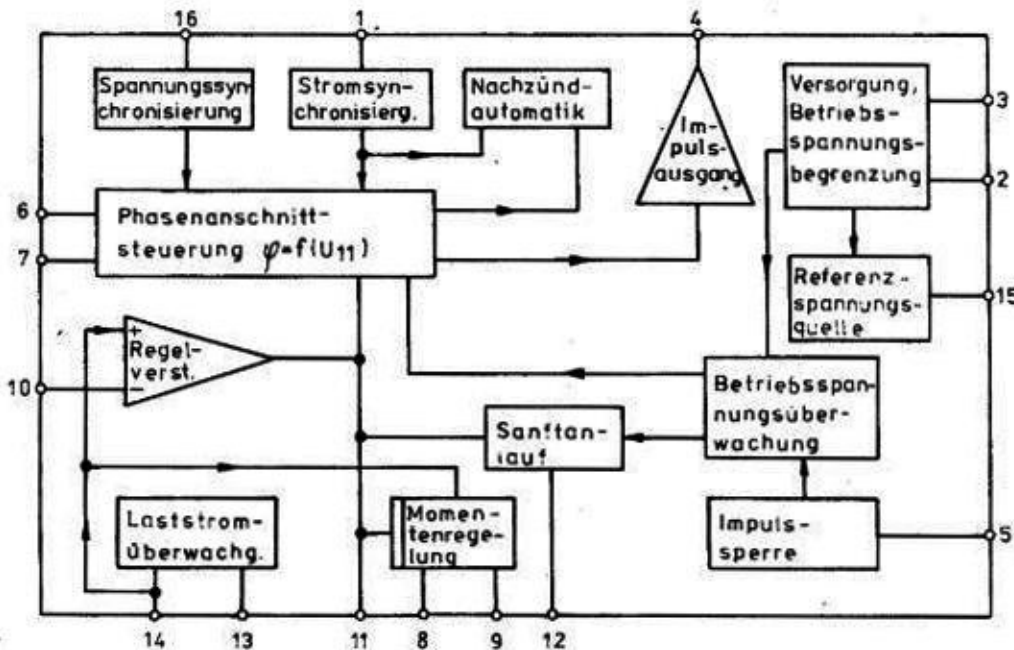
Bild 2: Blockschaltbild
