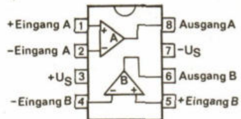
Doppel-OPV
