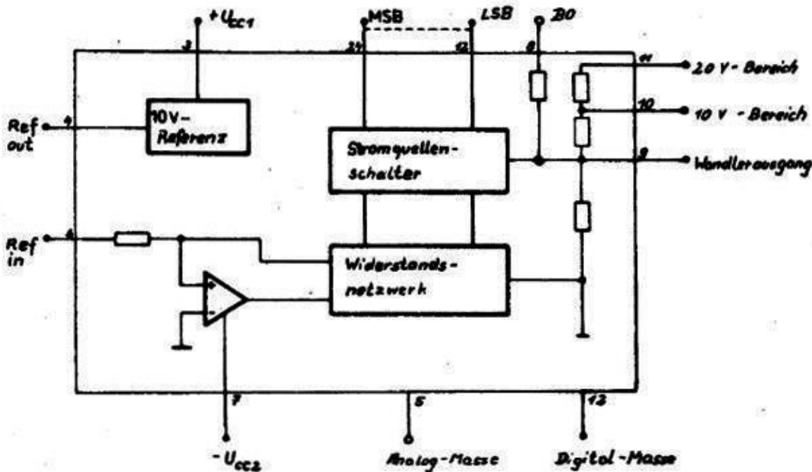
Bild 2: Blockschaltbild
