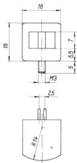
Maßskizze
