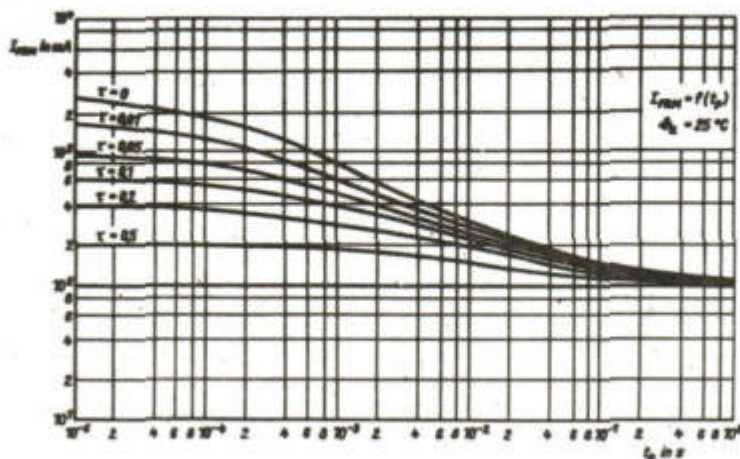
Bild 5: Impulsbelastungsdiagramm für den Spitzenstrom der Eingangsdiode und der Umgebungstemperatur \theta_a = 25 \text{ }^{\circ}\text{C} Parameter: \tau = \frac{t_p}{T}
