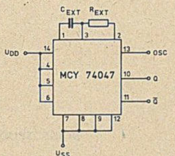
Multiwibrator astabilny
