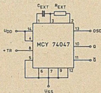
Multiwibrator monostabilny
