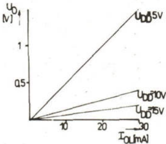
Funktion Ausgangsspannung/ Ausgangsstrom I_{OL}
