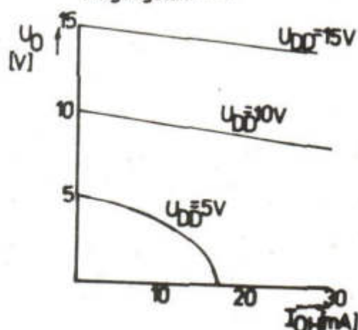
Funktion Ausgangsspannung/ Ausgangsstrom I_{OH}
