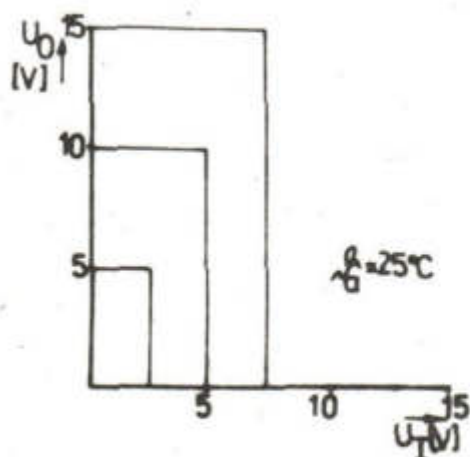
Übertragungsfunktion
