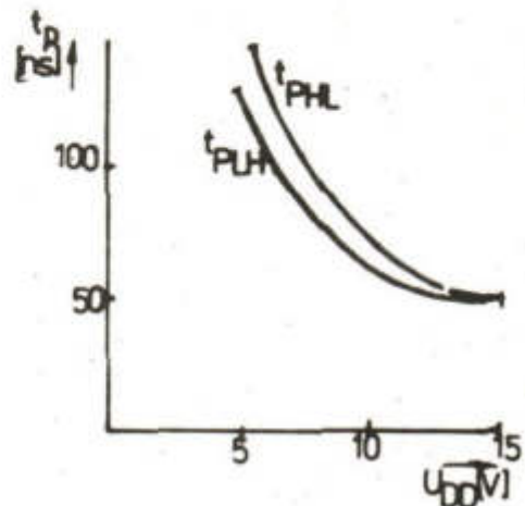
Funktion Gatterlaufzeit/ Betriebsspannung U_{DD}
