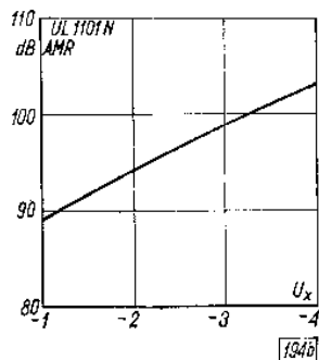
Współczynnik tłumienia sygnału wspólnego w funkcji napięcia polaryzacji U_x i układ pomiarowy
