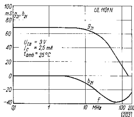
Kaskoda. Admitancja przejściowa w funkcji częstotliwości
