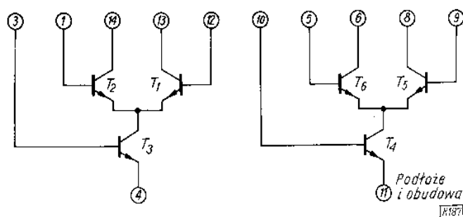
Schemat elektryczny
