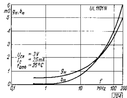
Kaskoda. Admitancja wejściowa w funkcji częstotliwości
