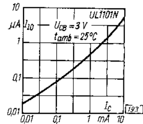
Prąd wejściowy niezrównoważenia w funkcji prądu kolektora
