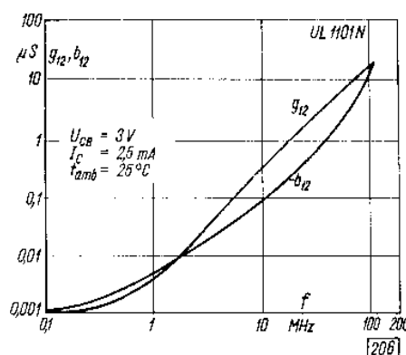
Kaskoda. Admitancja zwrotna w funkcji częstotliwości
