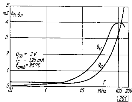
Wzmacniacz różnicowy. Admitancja wejściowa w funkcji częstotliwości
