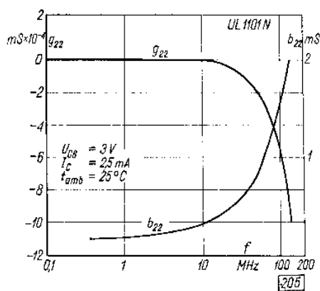
Kaskoda. Admitancja wyjściowa w funkcji częstotliwości
