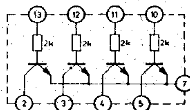
Schemat wewnętrzny
