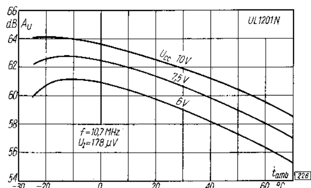
Wzmocnienie napięciowe w funkcji temperatury otoczenia
