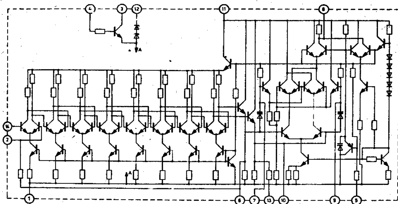
Schemat wewnętrzny
