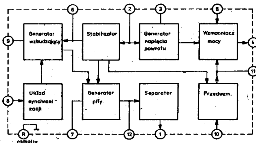
Schemat blokowy
