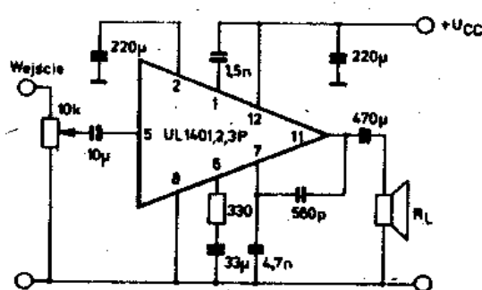
Schemat aplikacyjny
