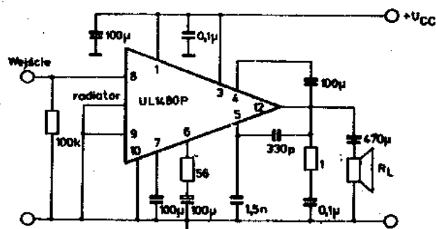
Schemat aplikacyjny
