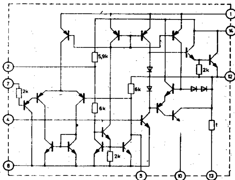
Schemat wewnętrzny
