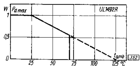
Dopuszczalna moc strat w funkcji temperatury otoczenia
