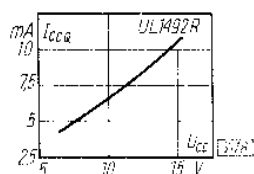
Prąd spoczynkowy zasilania w funkcji napięcia zasilania
