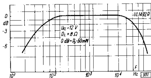
Wzmocnienie napięciowe w funkcji częstotliwości
