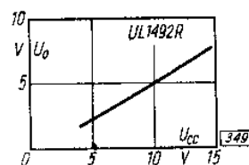
Napięcie spoczynkowe wyjściowe w funkcji napięcia zasilania
