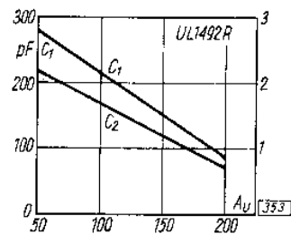
Pojemności C_1 i C_2 w funkcji wzmacnienia napięciowego
