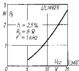
Moc wyjściowa w funkcji napięcia zasilania
