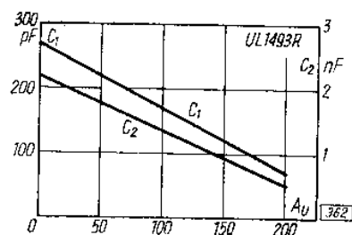
Pojemności C_1 i C_2 w funkcji wzmocnienia napięciowego
