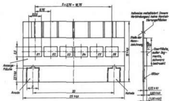
Bild 4: Maßbild VQH 604
