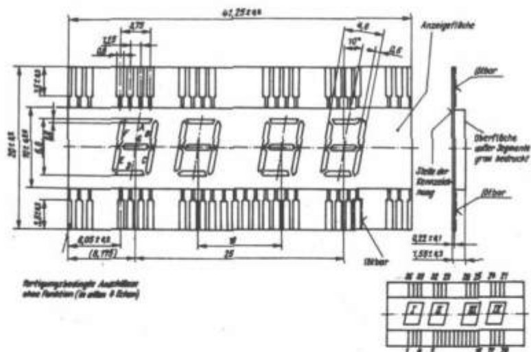
Bild 3: Maßbild VQH 207
