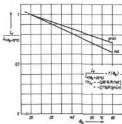
Bild 5: Relativer Temperaturkoeffizient der Lichtstärke VQH 205, VQH 206, VQH 207
