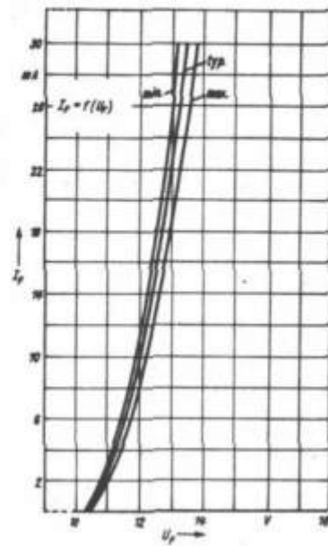
Bild 9: Durchlaßkennlinie VQH 604
