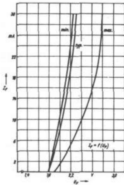
Bild 8: Durchlaßkennlinie VQH 205, VQH 206, VQH 207
